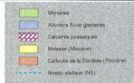
Extrait de l'étude hydrogéologique sur le périmètre du SAGE de la basse vallée de l'Ain (1999)
